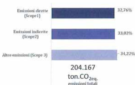
Figura 16: Emissioni di CO 2 eq.
